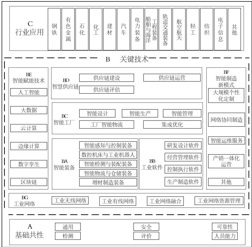
图 2 智能制造标准体系结构图
